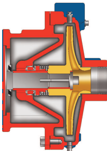
JM Motor 6BA Frame
