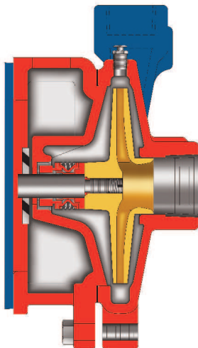
56J Motor 6B Frame
